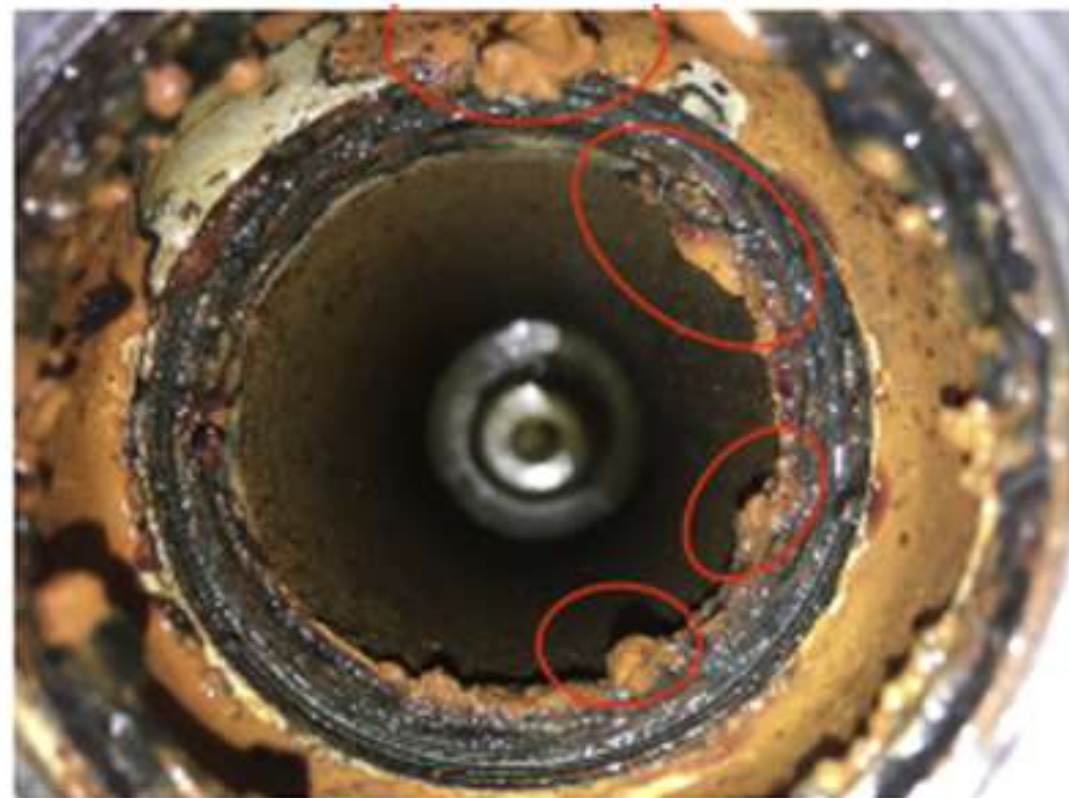
(左) NMR パイプテクター設置箇所よりも上流の配管 (右) NMR パイプテクター設置箇所よりも下流の配管
